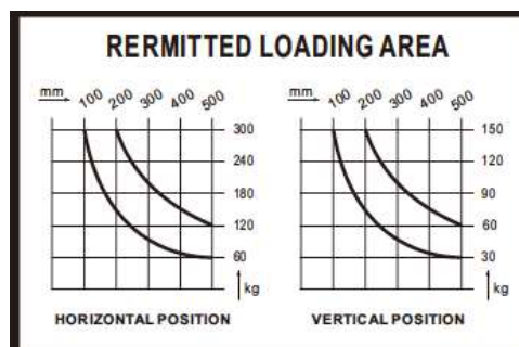
Diagram: ECO S300
